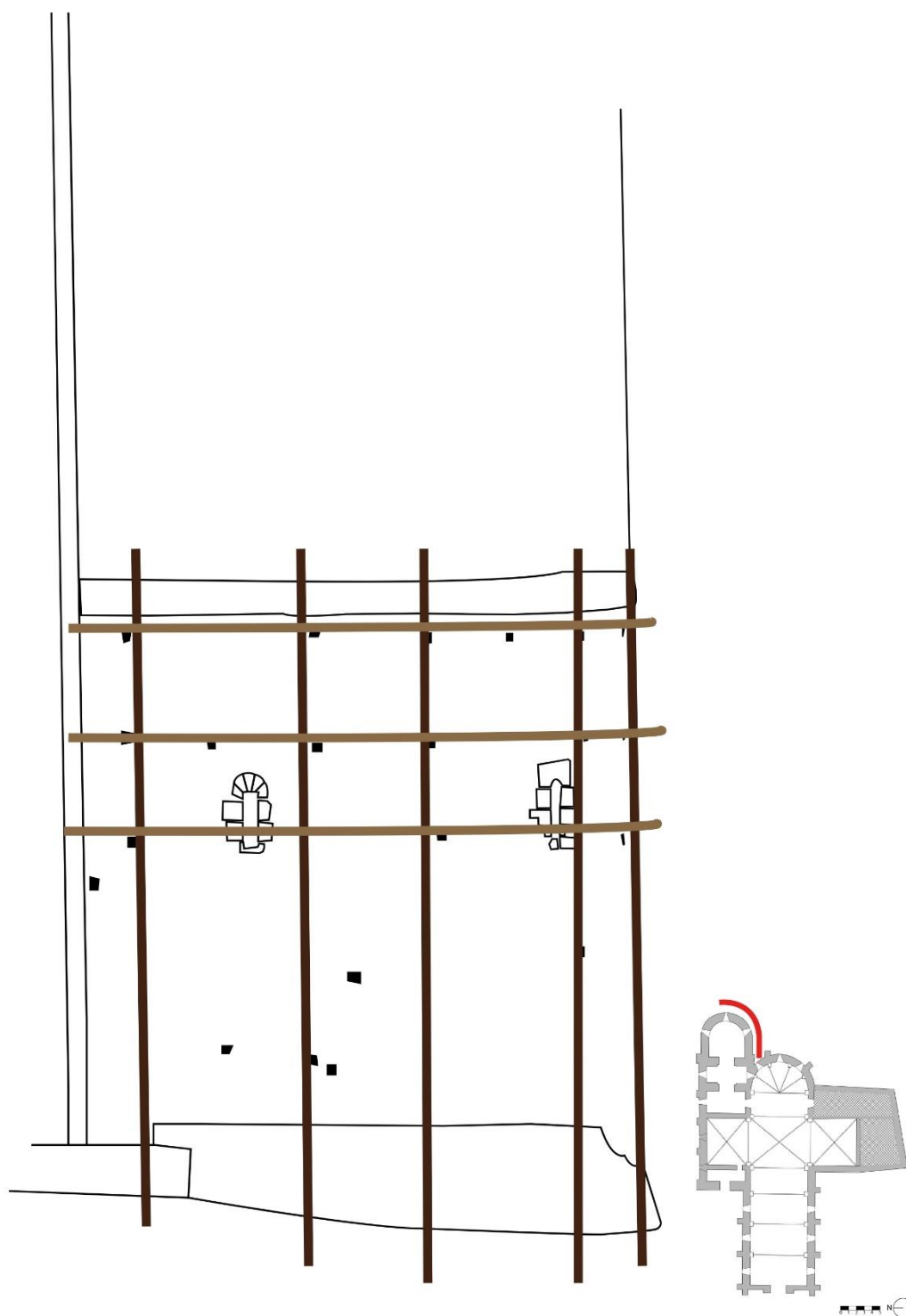
Figure 48 : Échafaudage restitué au niveau de l'abside côté sud
