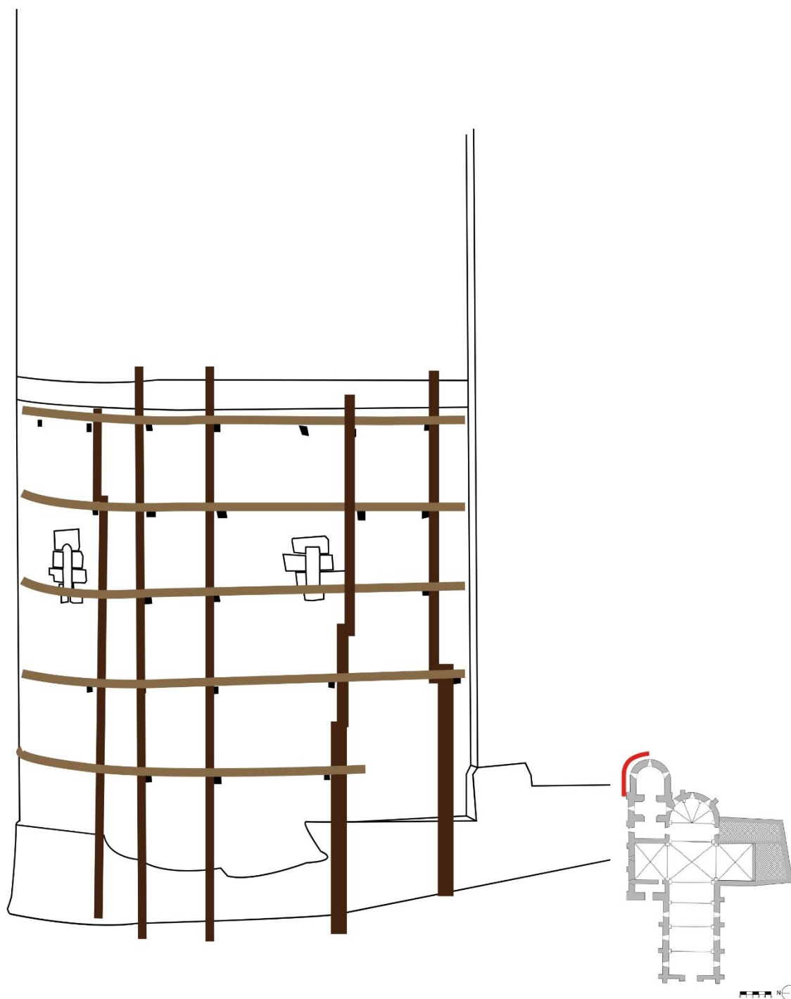
Figure 47 : Échafaudage restitué au niveau de l'abside côté nord
