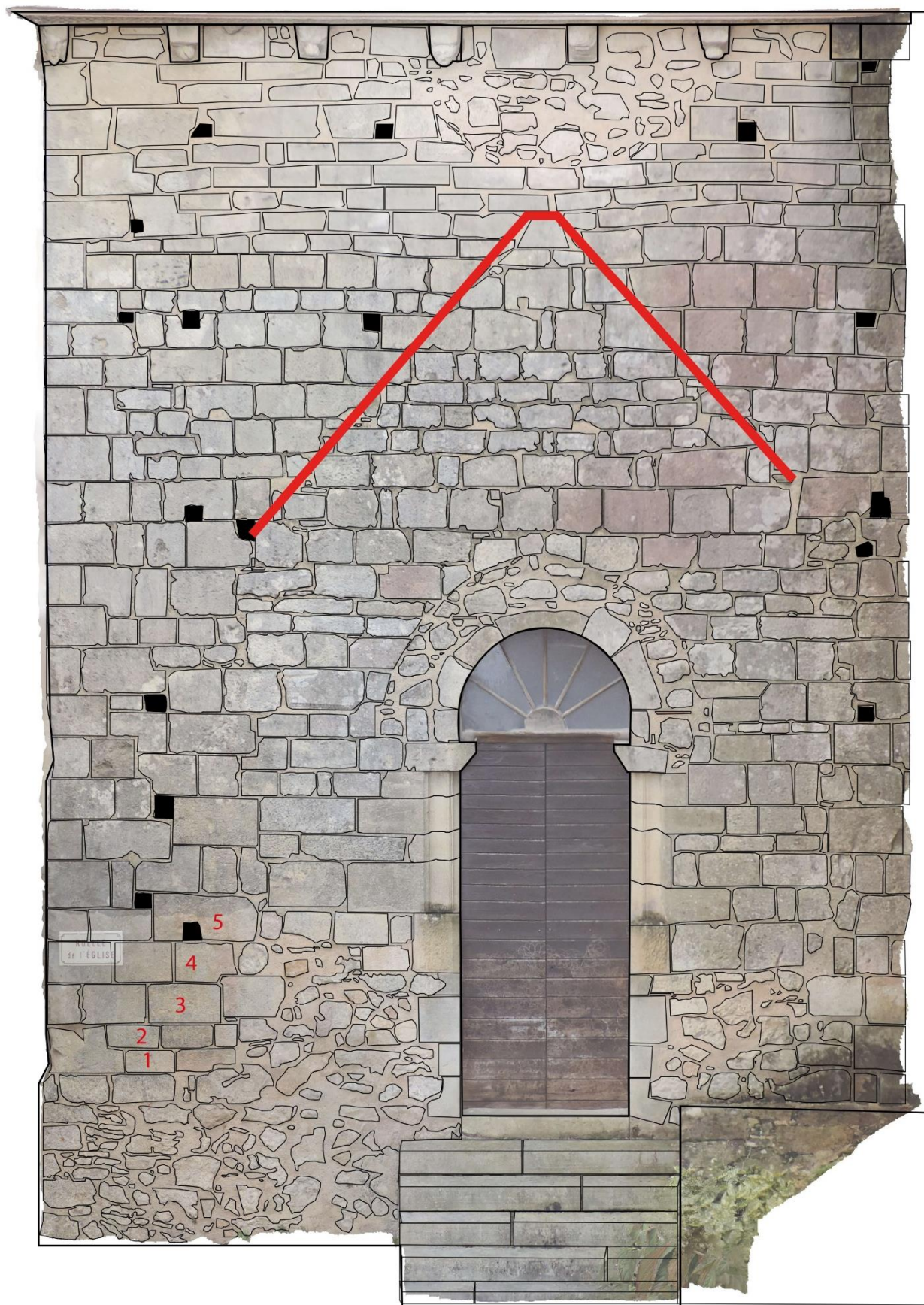
Figure 38 : Numérotation des blocs au-dessus de la ligne de fondations au nord de la façade romane occidentale
