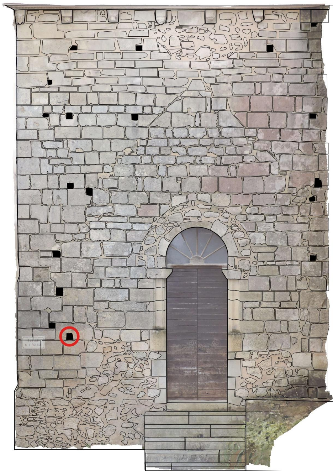
Figure 43 : Trou de boulin façonné au nord de la façade romane occidentale
