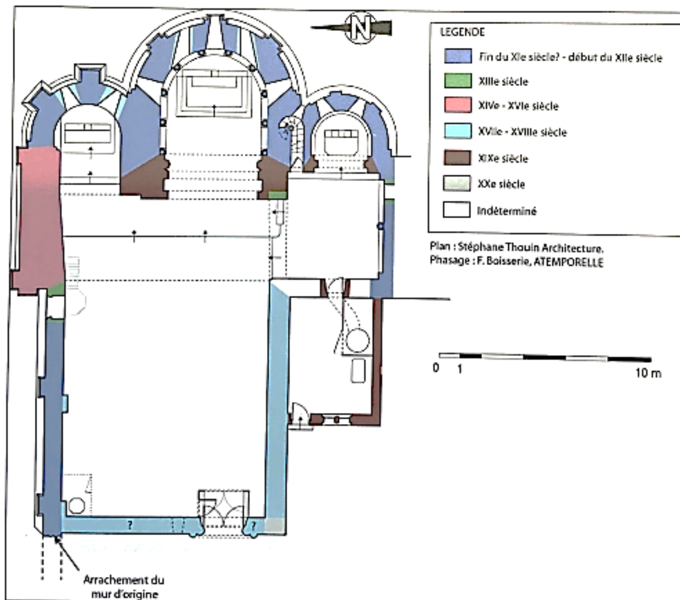
Figure 54 : Plan phasé issu du rapport consacré à l'église Saint-Front, DAO phasage réalisé par Florence BOISSERIE 1
