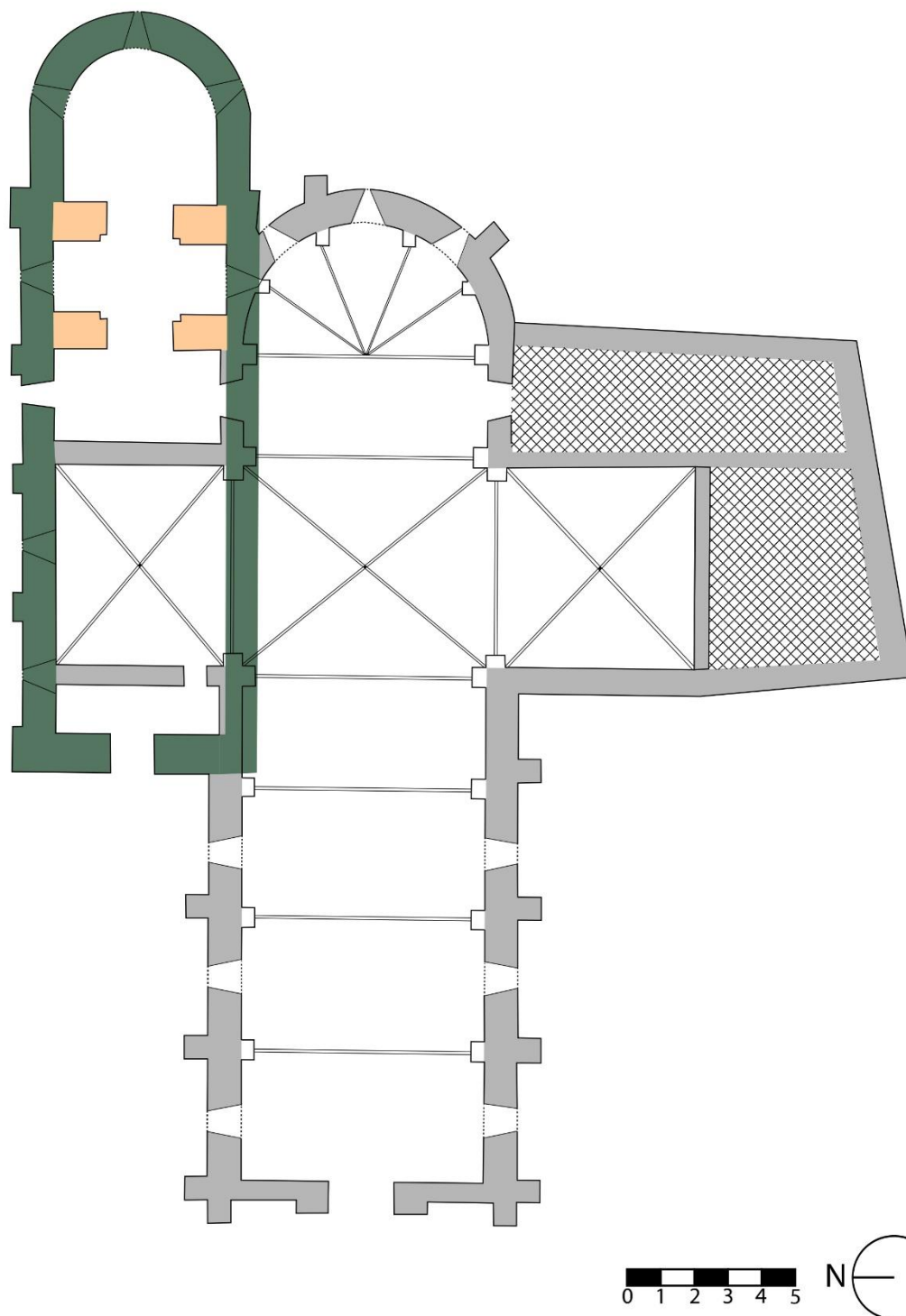
Figure 30 : Restitution du plan de l'église romane – Manon CAUCHI
