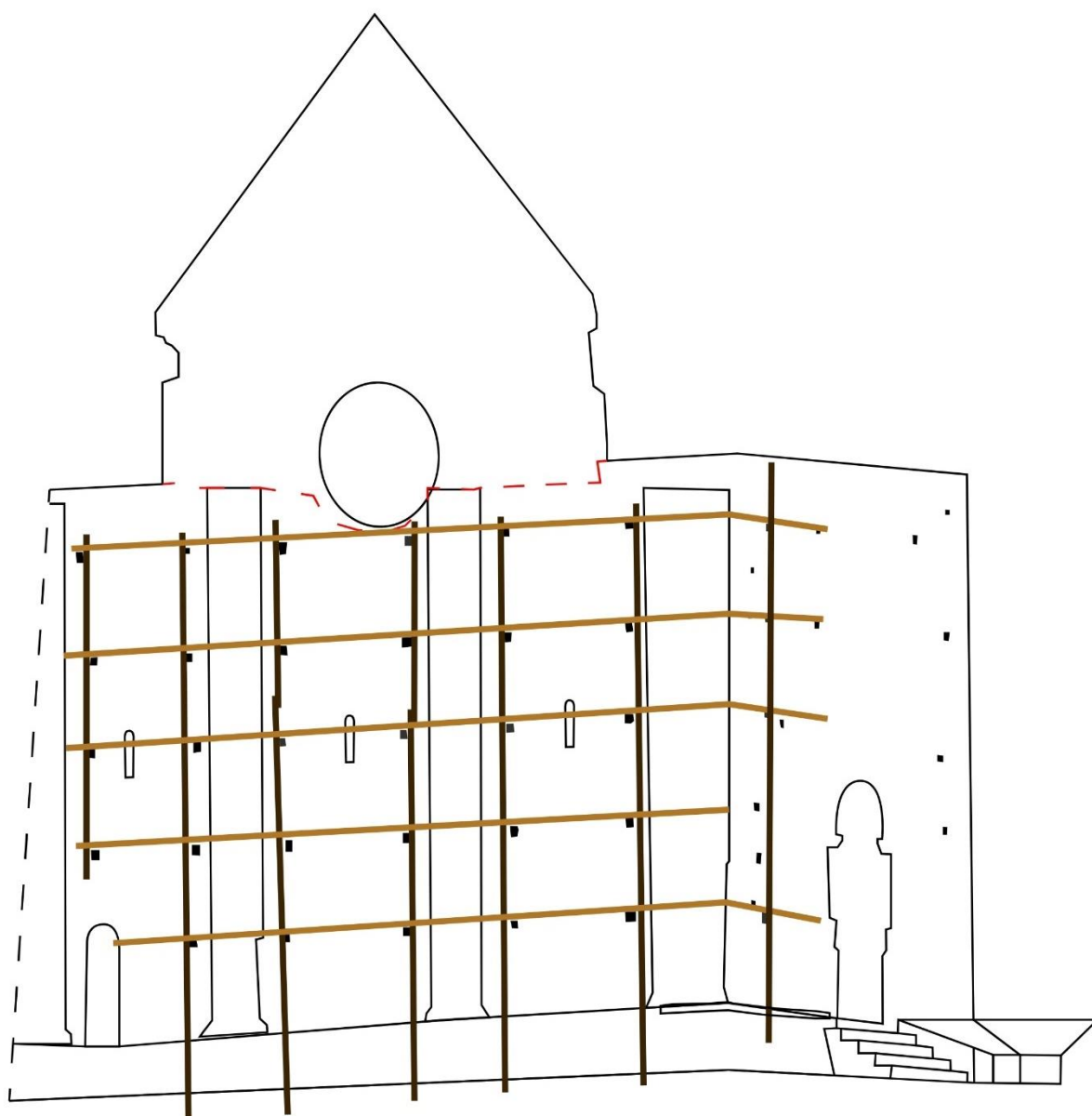
Figure 41 : Restitution des échafaudages à la jonction du mur nord et de la façade romane occidentale
