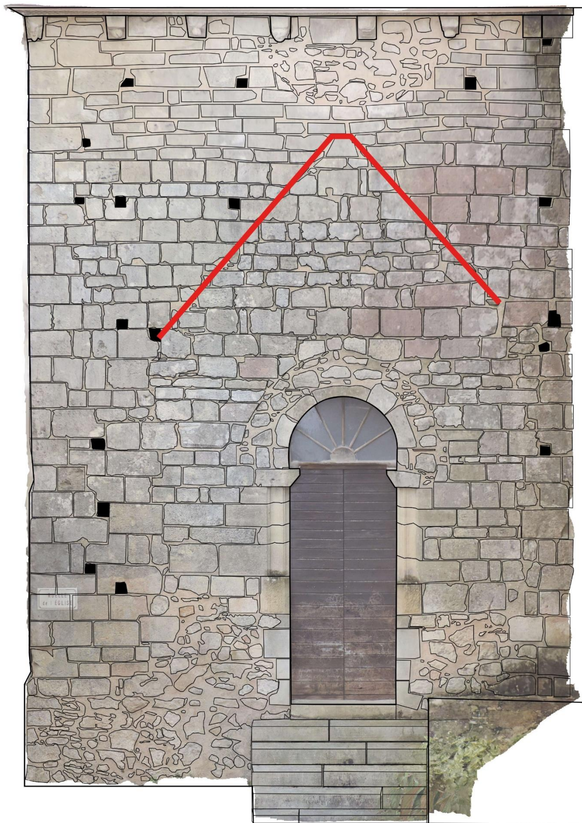
Figure 37 : Marque triangulaire sur la façade romane occidentale
