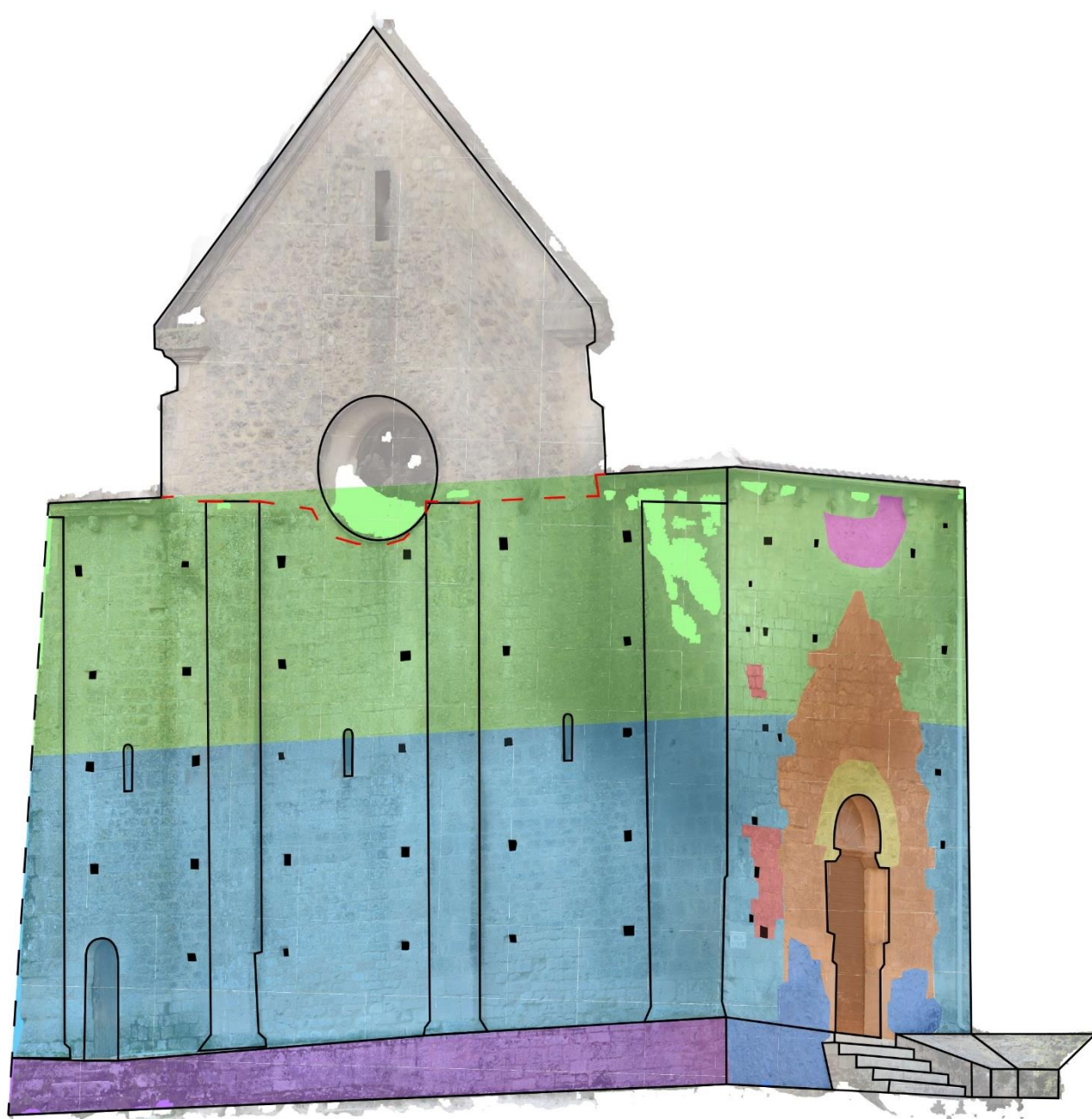
Figure 51 : Chronologie relative tendue sur le mur nord et sur la façade romane occidentale
