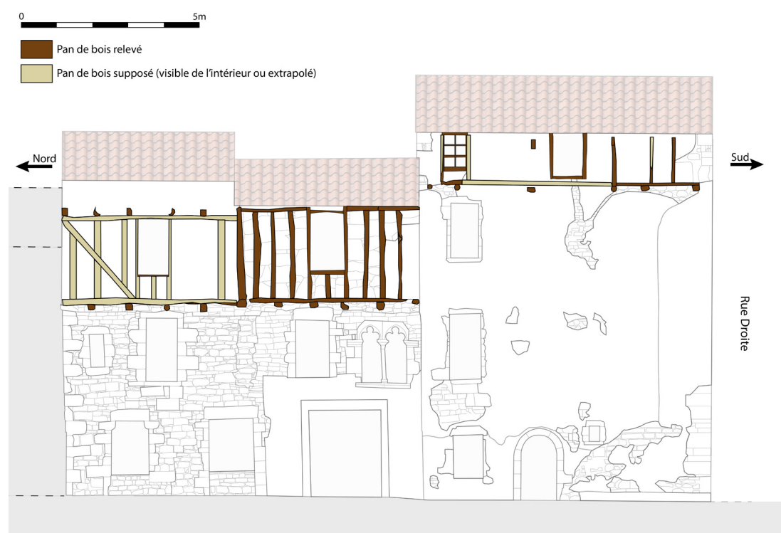
fig. 63 : relevé rue du Commandant Alibert, détail des pans de bois (Relevé et D.A.O. : Eric Chabanne)
