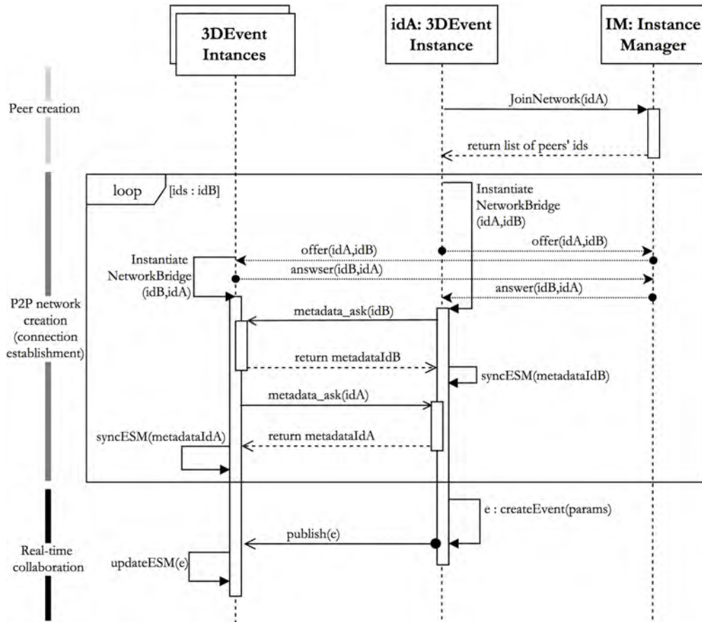
FIGURE 3.9 – Protocole de connexion au réseau d'instance 3DEvent
