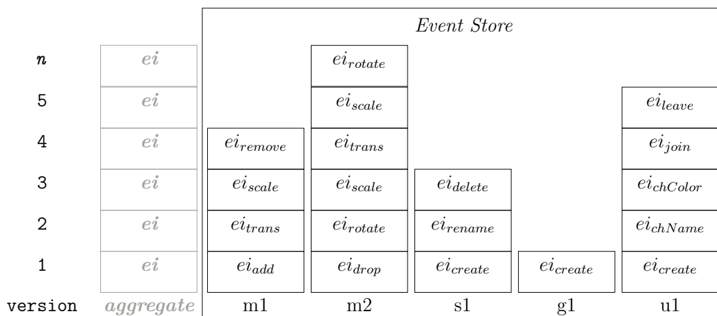
FIGURE 3.3 – Représentation d'un journal d'événement stockant des agrégats (« m1 », « m2 », « s1 », « g1 », « u1 ») versionnés (de 1 à n) qui contiennent des instances d'événements ( ei_{typeEvent} )
