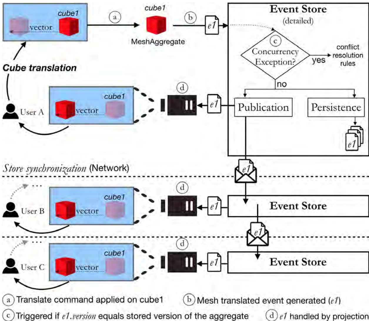
FIGURE 4.5 – Exemple d'édition collaborative où User A est connecté à User B, lui même connecté à User C. Le cycle montre les différentes étapes du déclenchement : la commande, la génération de l'événement, la synchronisation du journal d'événements, l'impact sur le rendu des autres utilisateurs pour une translation sur un cube et le rendu visuel.
