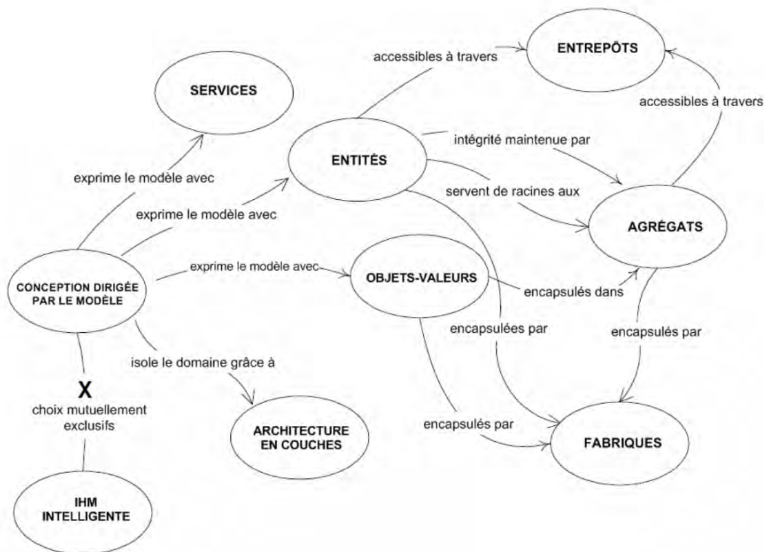
FIGURE 2.6 – Illustration du patron DDD et de ses artefacts (issue de [Avram et Marinescu, 2006] sous licence Creative Commons)
