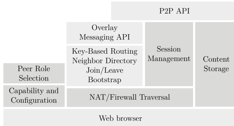
FIGURE 3.6 – Composants de chaque pair dans 3DEvent (point de vue réseau)
