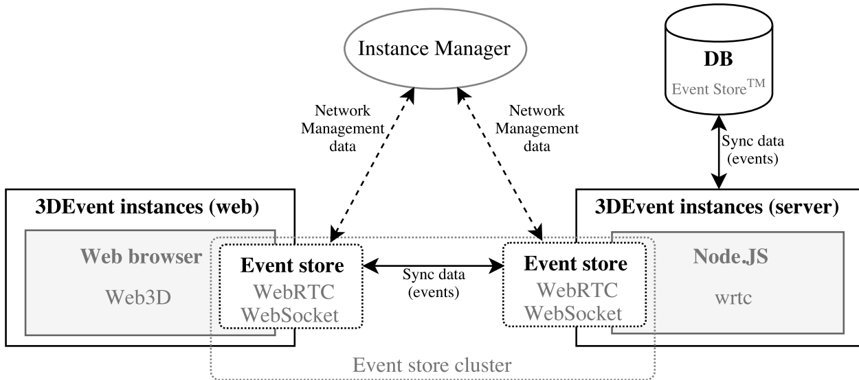
FIGURE 3.7 – Architecture de communication « orientée événements »
