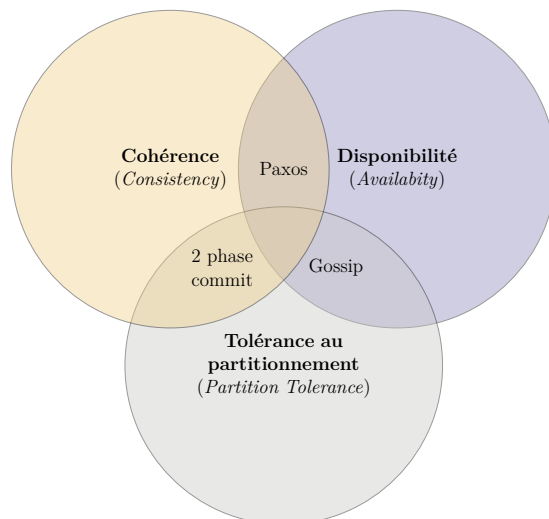
FIGURE 3.4 – Théorème CAP et les algorithmes de compromis
