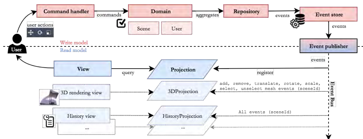
FIGURE 3.2 – Modèle de l'architecture client dans 3DEvent : la gestion du cycle de vie des données avec CQRS et ES dans un navigateur web, des actions des utilisateurs à la visualisation en passant par la synchronisation réseau.
