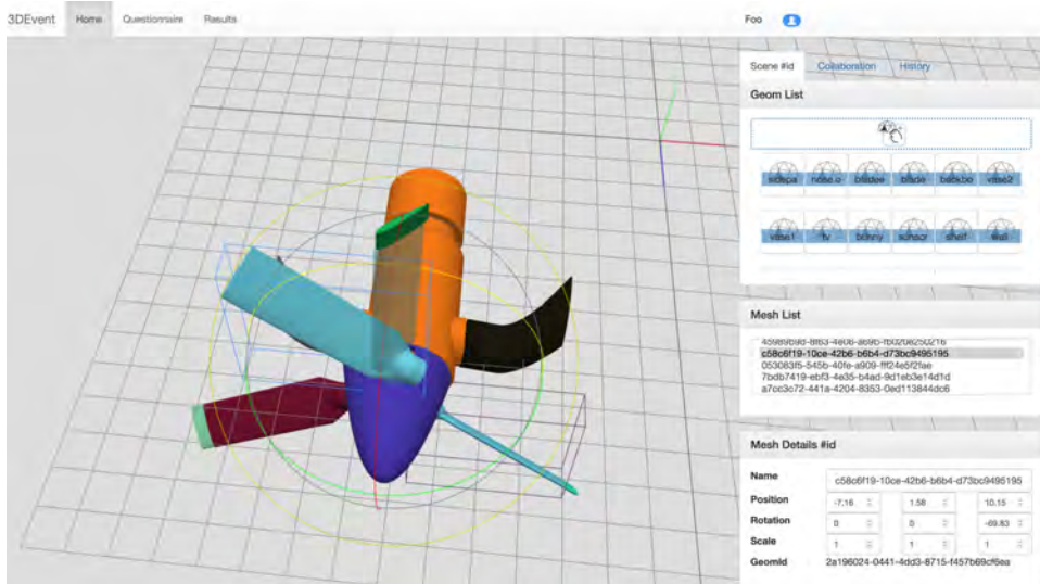
(a) Rotation (environnement 3D) et outils pour la manipulation d'objet 3D (panneau latéral)
