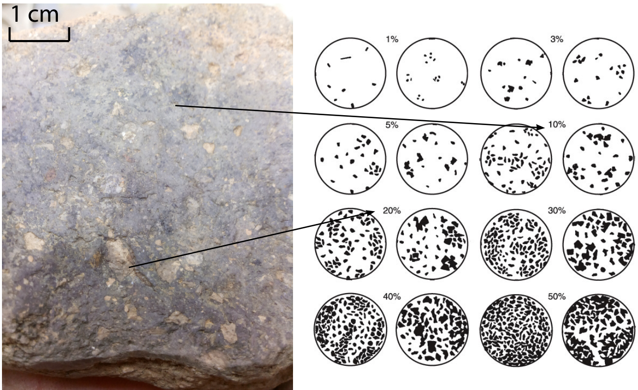
Annexe 36 - Comparaison de la proportion de dégraissant de chamotte avec l'échelle graphique de Terry et Chilingar (Terry et Chilingar, 1955).
