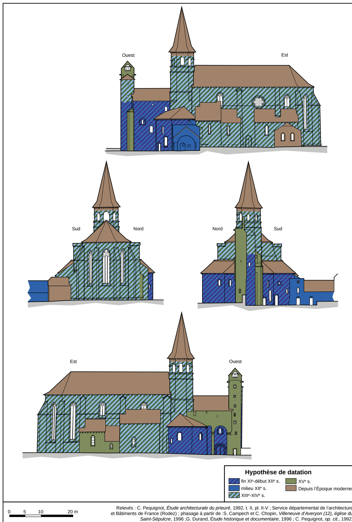
Fig. II-31 : Élévations de l'église du Saint-Sépulcre et proposition de phasage.
