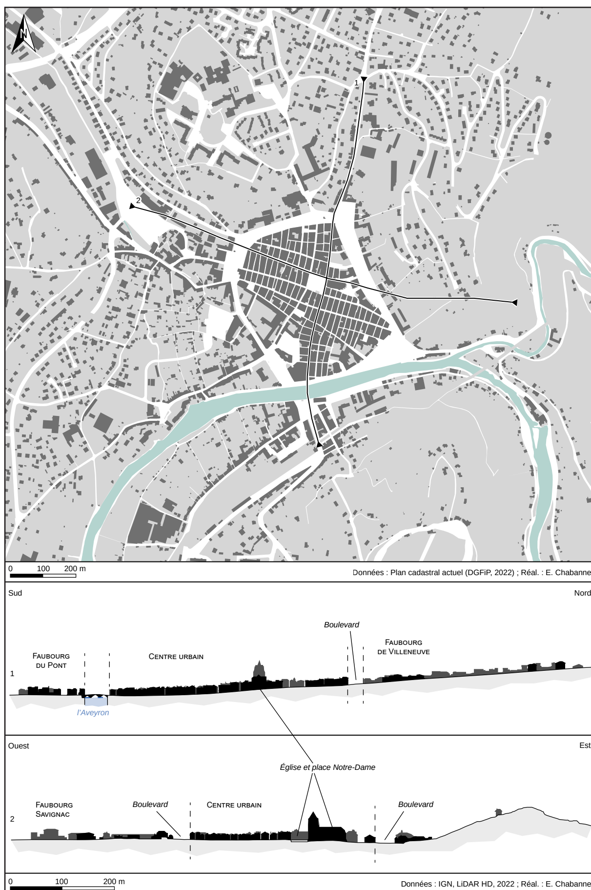
Fig. III-27 : Coupes topographiques de l'agglomération.
