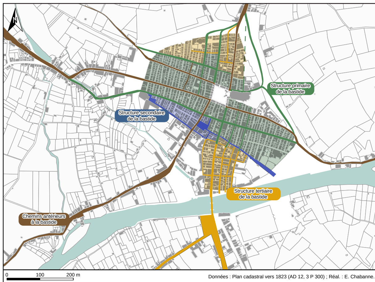
Fig. III-26 : Caractérisation de la structure de la bastide de Villefranche.
