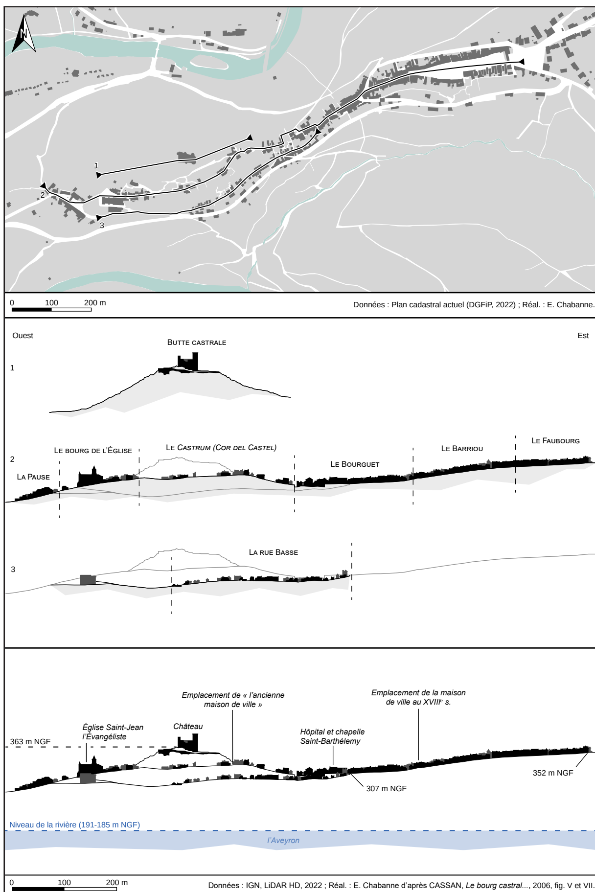
Fig. I-25 : Coupes topographiques de l'agglomération.
