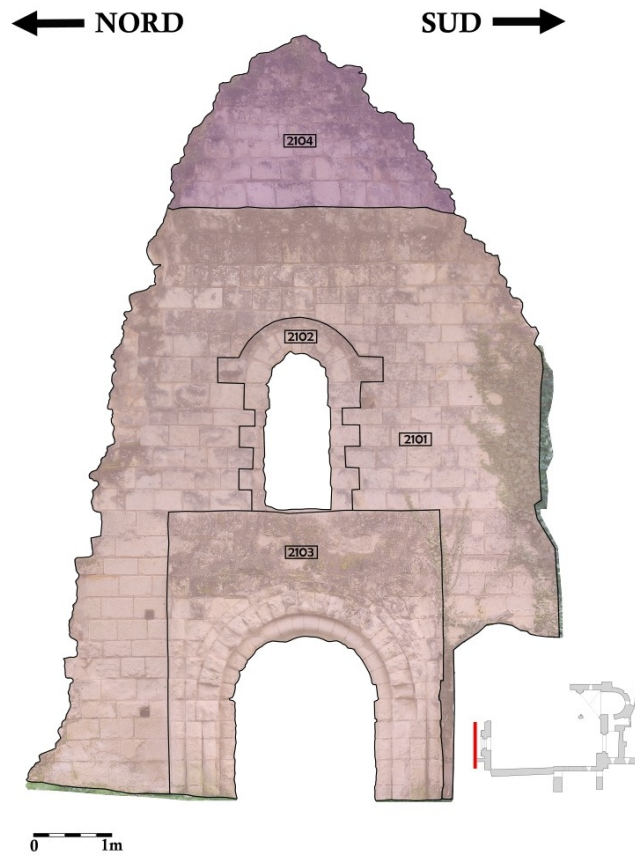
[Figure. 24] Répartition des unités construites sur l'orthophotographie de la face extérieure du pignon occidental de l'église Saint-Maxenceul à Cunault.
